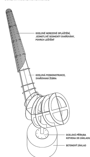
SCHEMA NOSNÉ KONSTRUKCE
