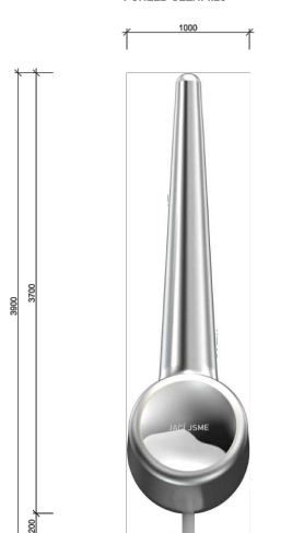
POHLED ČELNÍ 1:20
