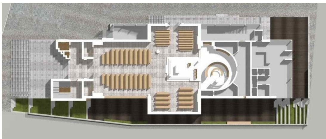
Půdorys areálu kostela a komunitního centra na Barrandově
